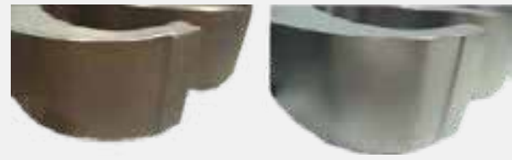
Oberfläche vor und nach dem Beizen mit POLINOX TB 100, Abtrag 70 µm
